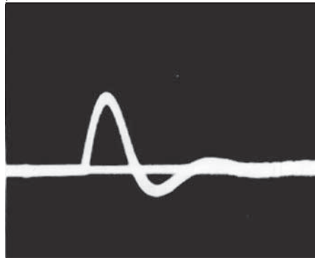
Obrázek 1. Oscilogram prahového defibrilačního impulsu – kondenzátorový impuls vedený přes indukci
