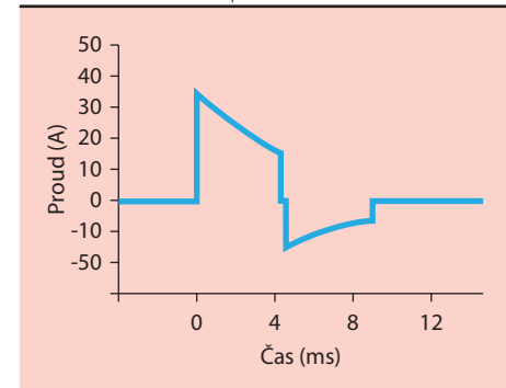
Obrázek 5. Průběh proudu při bifázickém rektilineárním výboji
