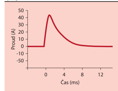
Obrázek 4. Znázornění průběhu proudu u bifázického truncated exponenciálního defibrilátoru
