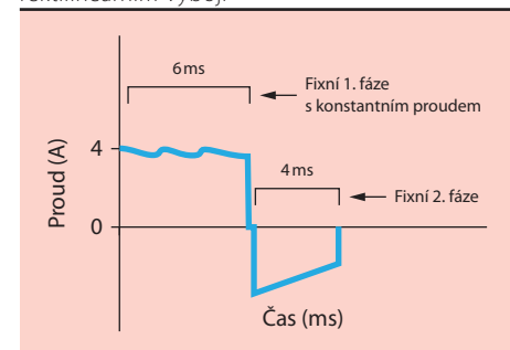
Obrázek 5. Průběh proudu při bifázickém rektilineárním výboji
