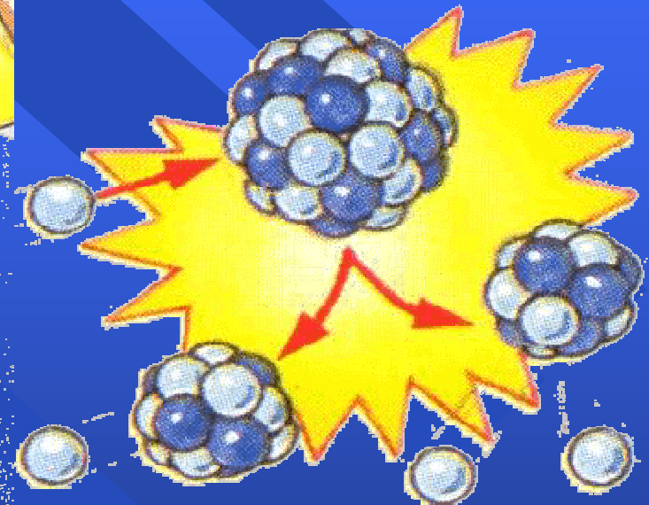
Jaderné štěpení
