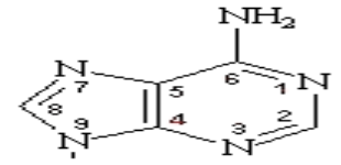
adenin
