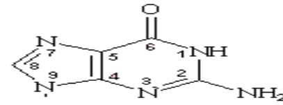
guanin
