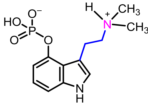
Psilocybin
