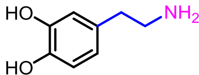
Dopamine
