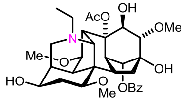
Aconitine
