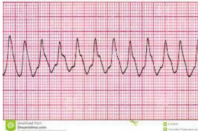
Ventricular Tachycardia
